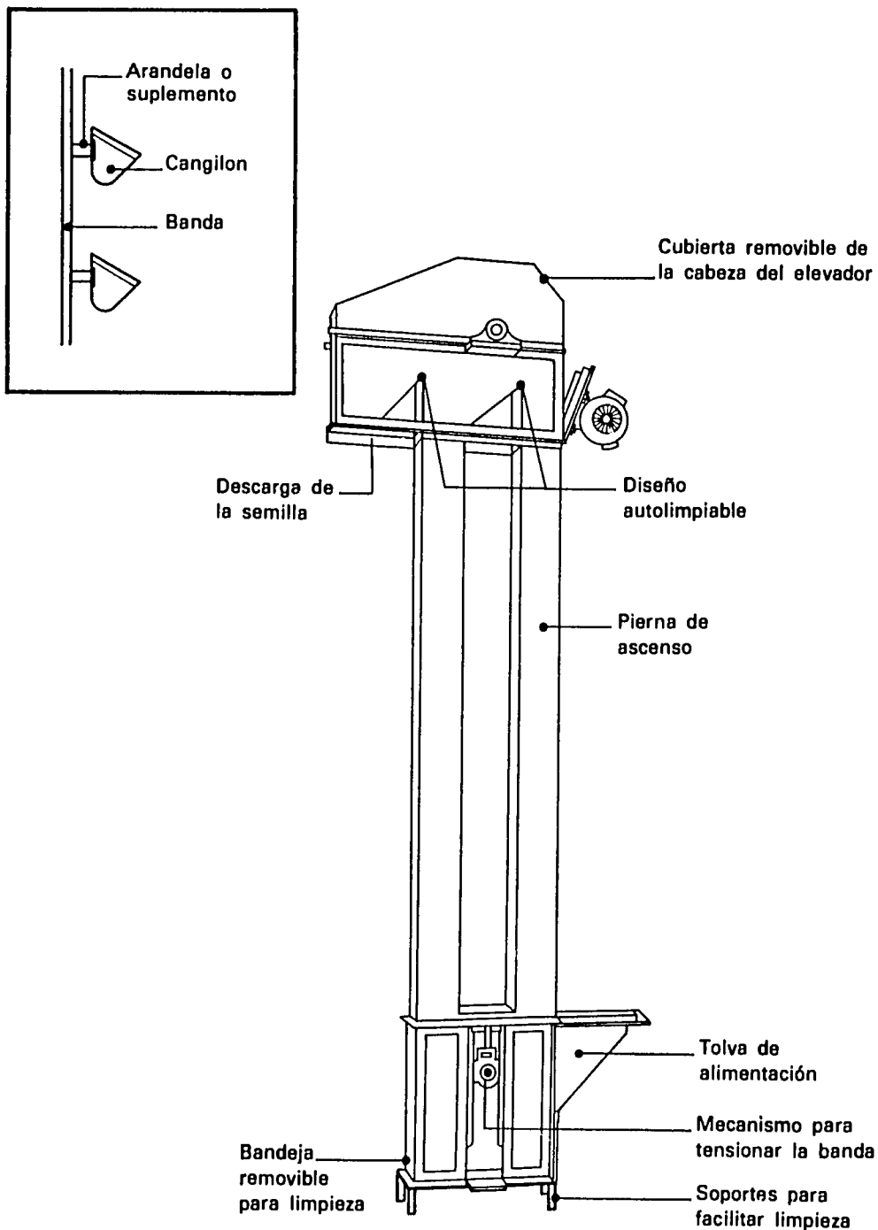
Figura 18. Detalles importantes para el diseño de un elevador de cangilones para semillas.
