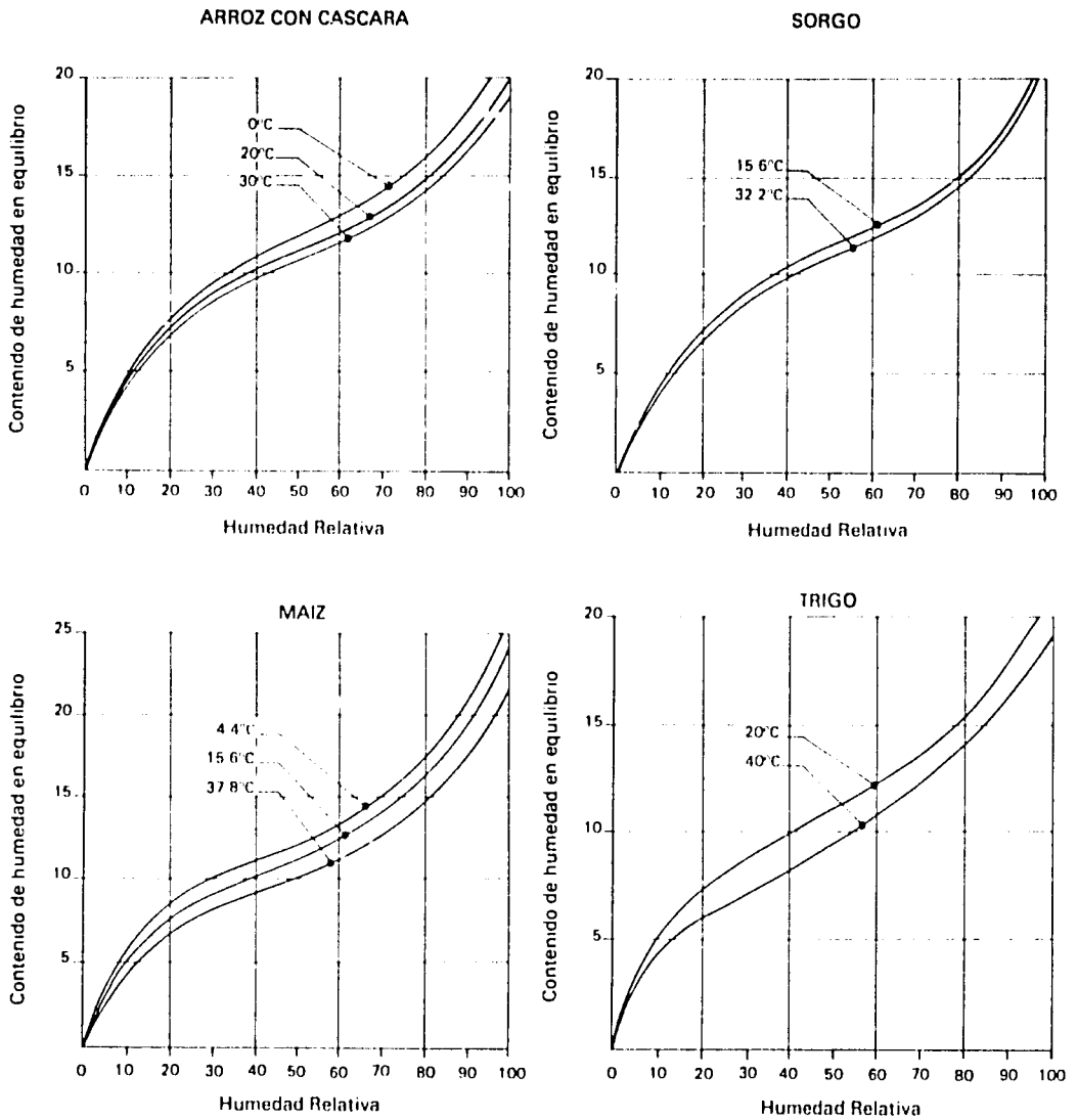
Figura 4. Curvas de contenido de humedad en equilibrio calculadas con la ecuación de Roa.
