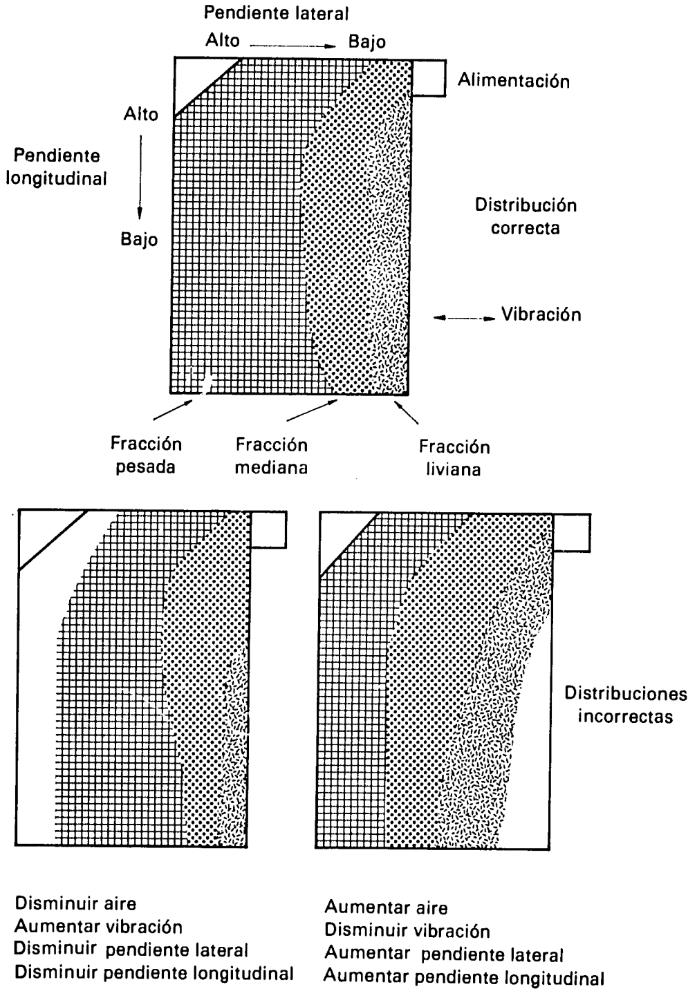
Figura 16. Distribución del material en la plataforma de la mesa de gravedad.)
