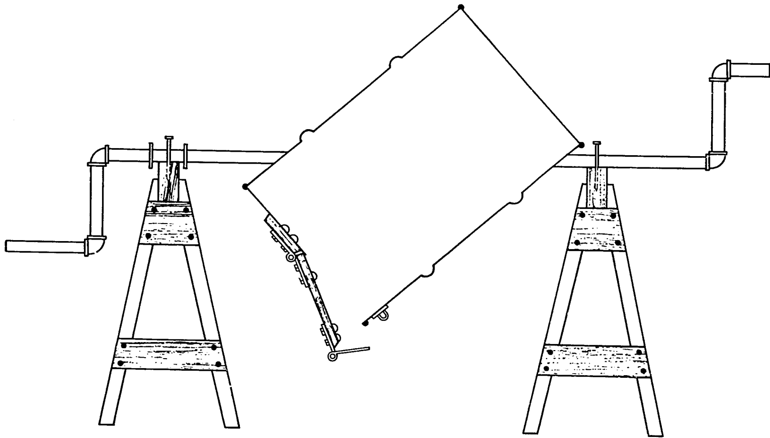
Figura 17. Tratadora manual.
