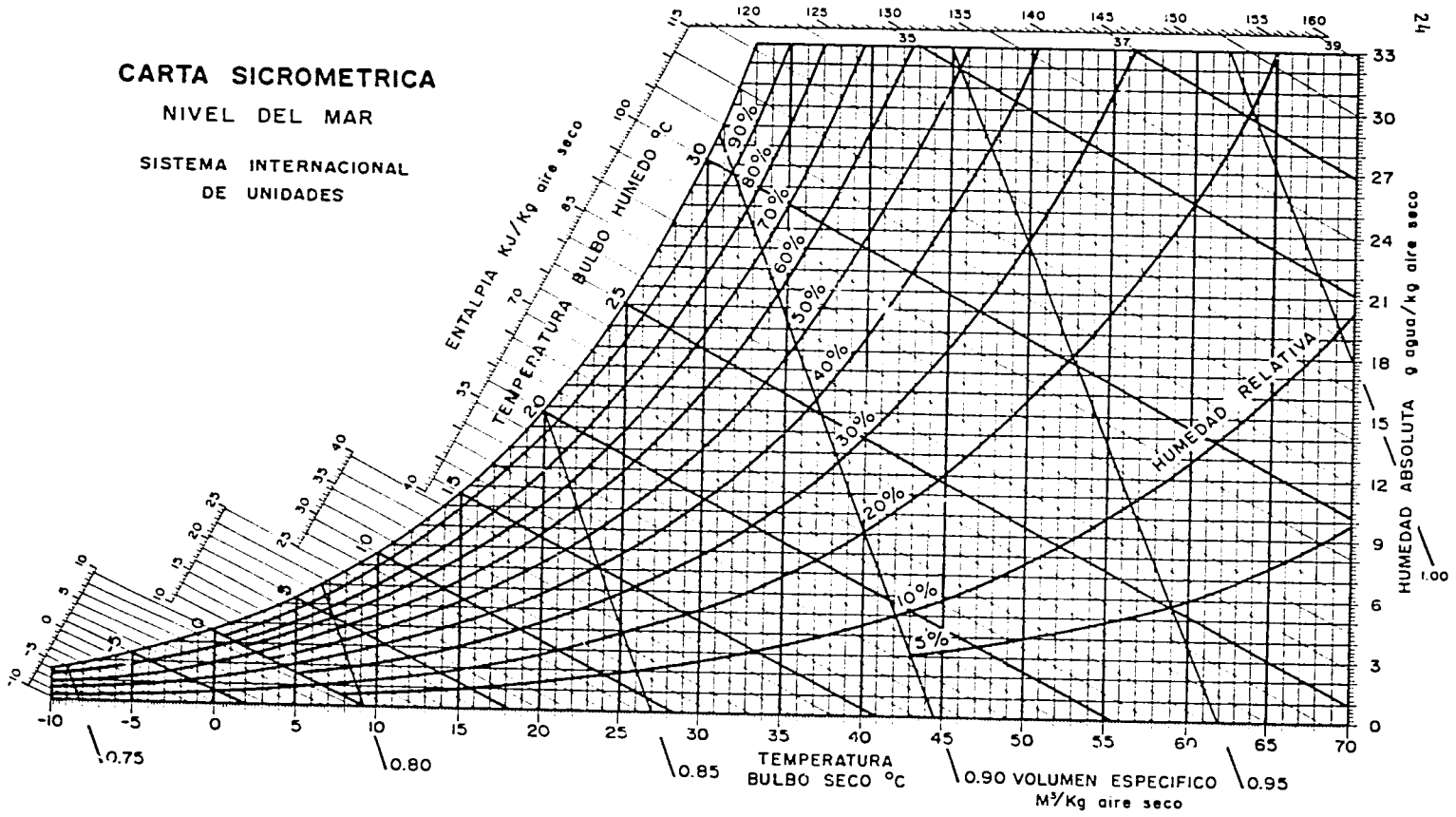
Figura 11. Carta sicrométrica.
