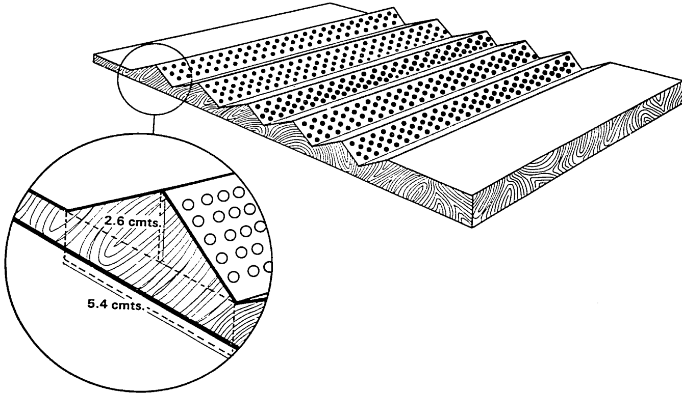
Figura 15. Zaranda ondulada.
