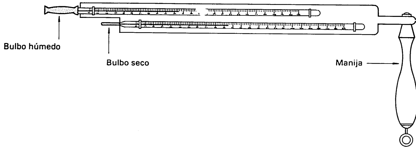
Figura 12. Sicrómetro de voleo.
