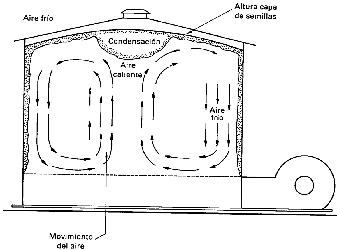
Figura 20. Migración de humedad en un silo de almacenamiento.
