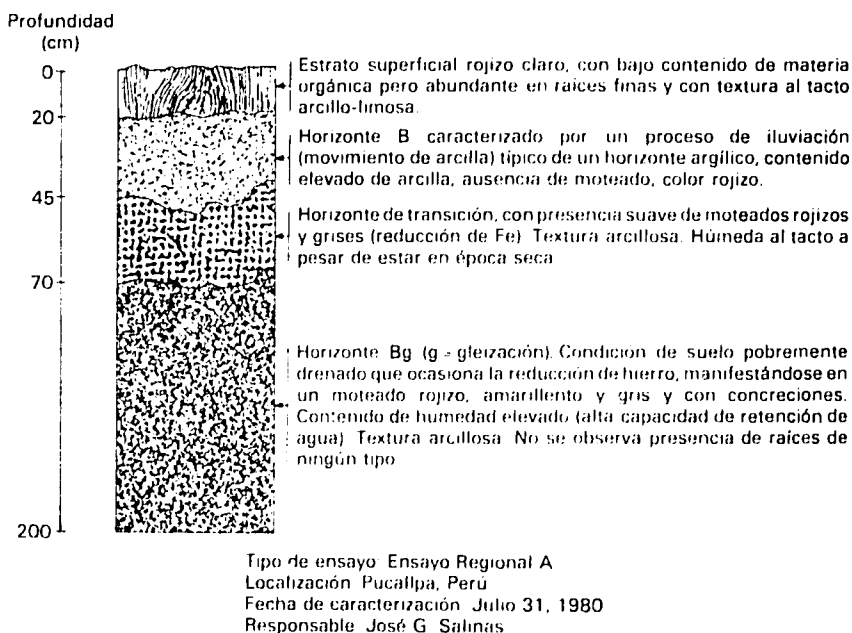
Figura 3. Ejemplo de una descripción general del perfil del suelo.
