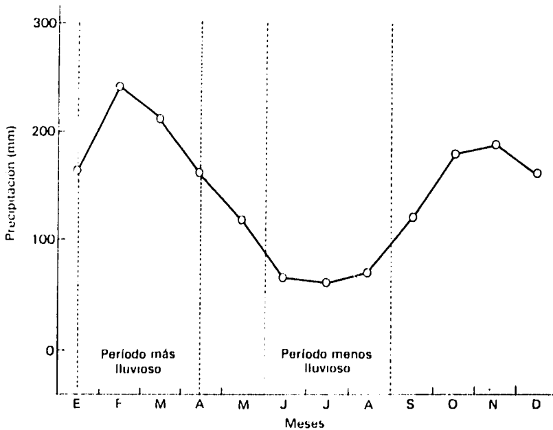
Figura 7. Ejemplo de selección de los períodos de máxima y mínima precipitación, según la distribución de las lluvias registras en años anteriores en un lugar de la Amazonia ( \bar{X} 20 años).
