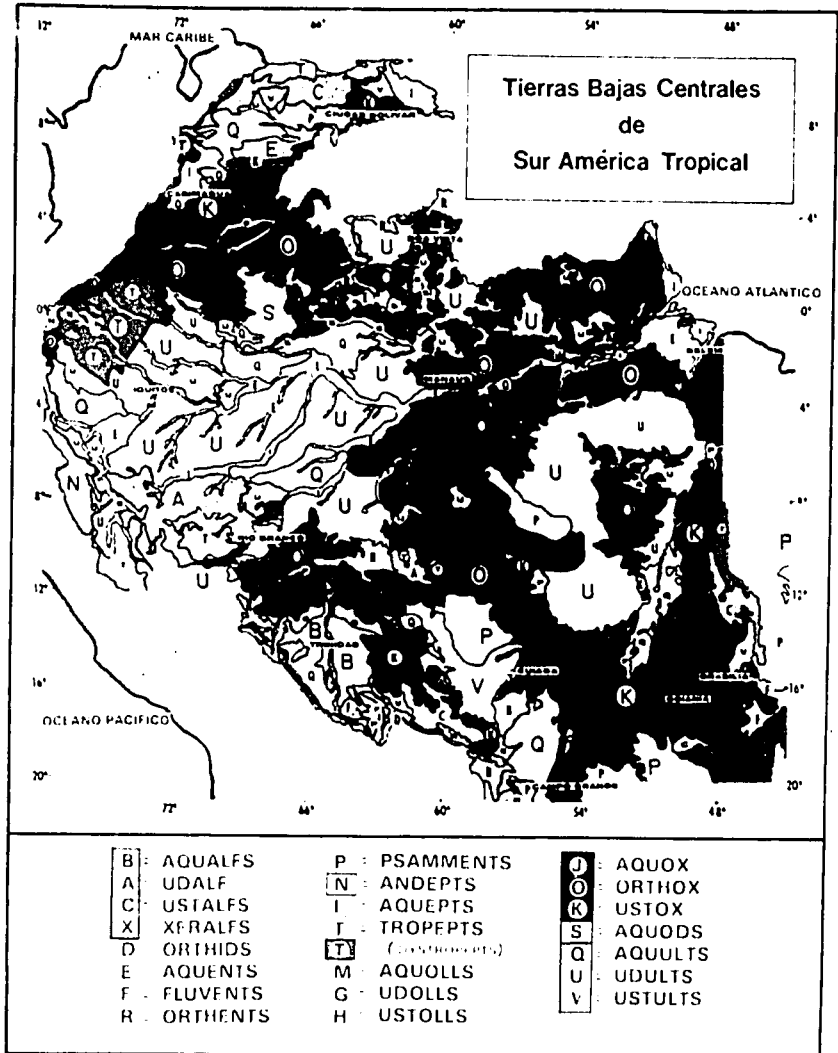
Figura 7 Mapa de las clases de los subórdenes del suelo que muestra los suelos con posibles cargas variables
