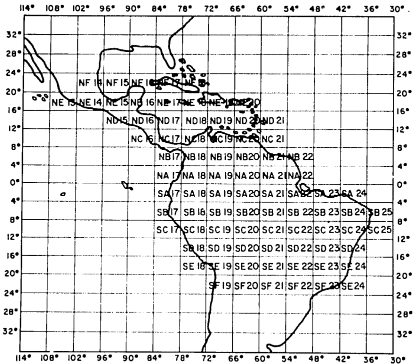
Figura 1. Cobertura del mapa del CIAT del sistema de tierra en las tierras bajas de América del Sur tropical. Los códigos (numero y letra) son los del Índice usado para el Mapa Mundial a la escala 1:1.000.000
