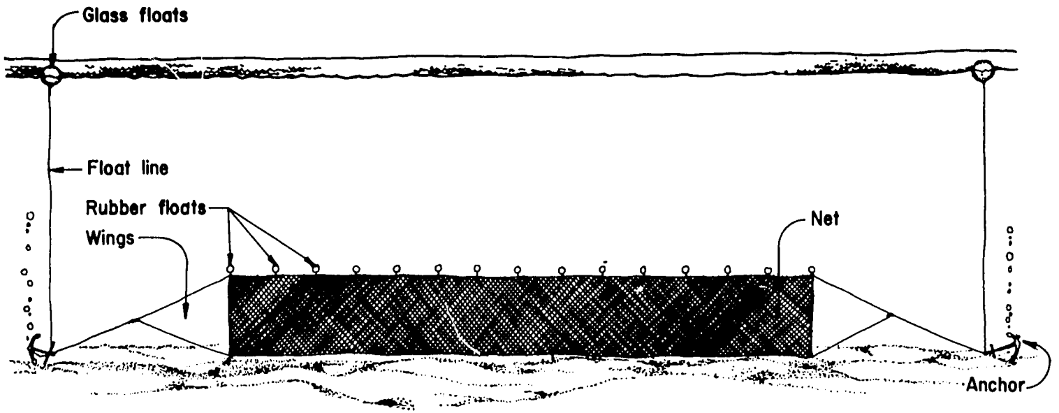
Fig. 11. A bottom set gill net.
