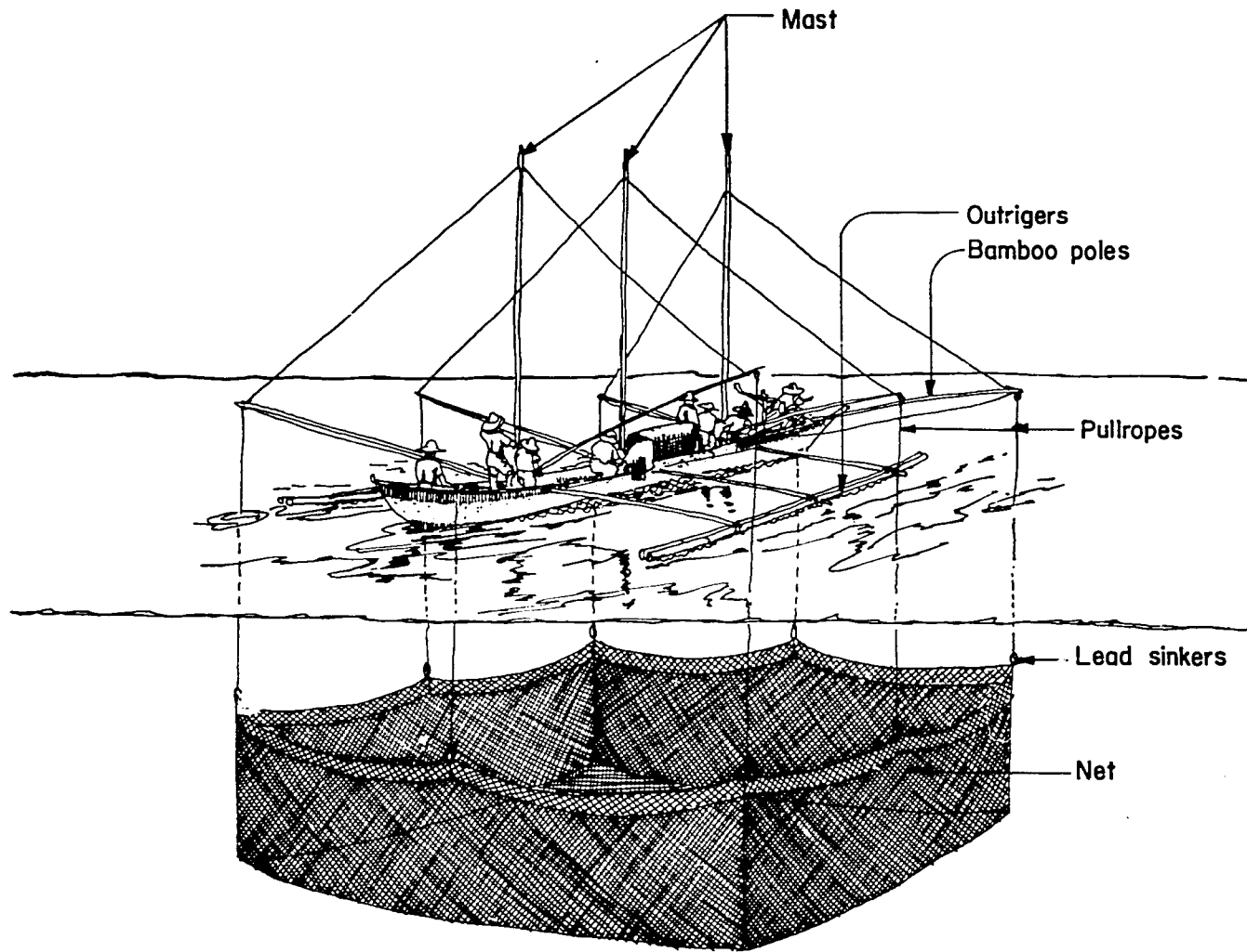
Fig. 14. Basnig (Pilipino), a typical bag net.
