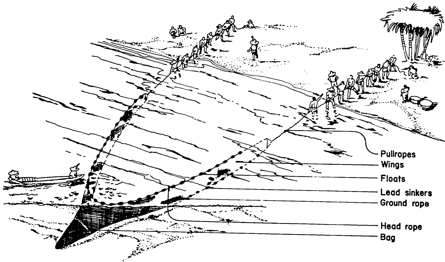
Fig. 15. Pukot (Pilipino), a typical beach seine.
