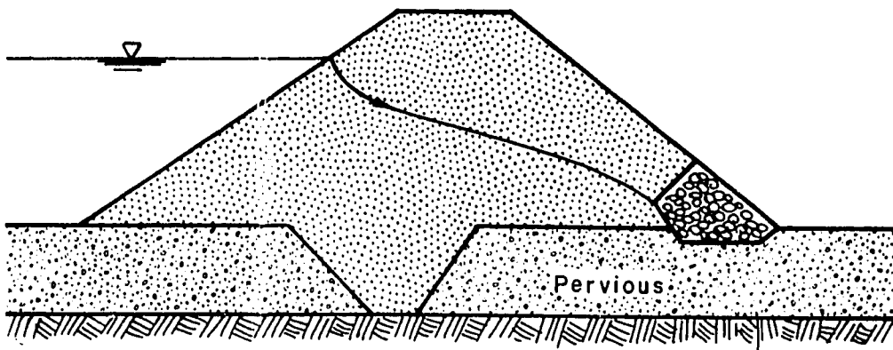
(d) Pervious with Cutoff and Drain
